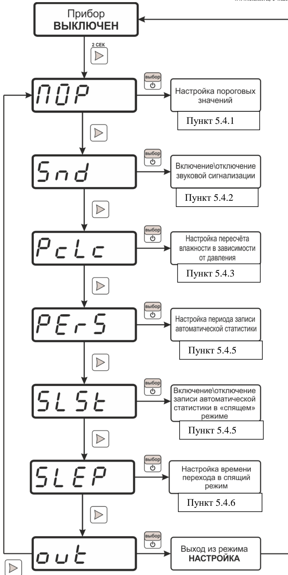
Рисунок 5.2 Схема режима НАСТРОЙКА ИВГ-1 К-П
