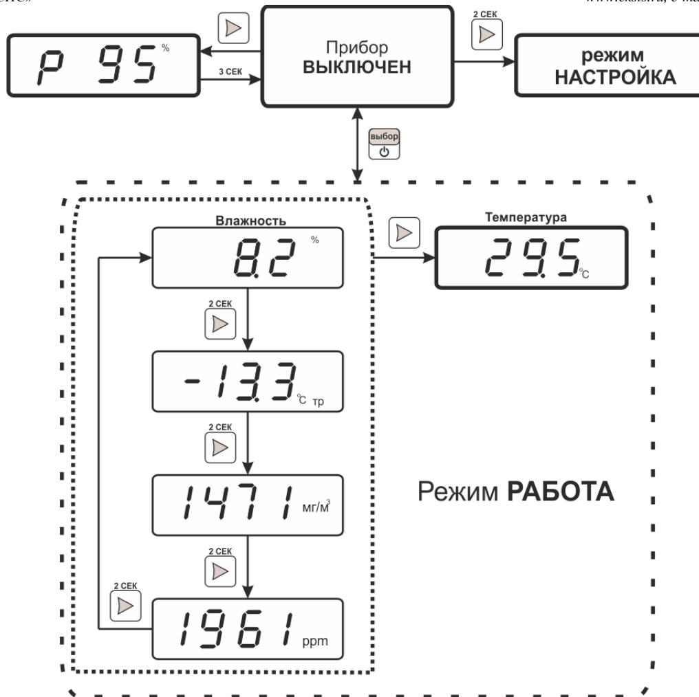
Рисунок 5.1 Режим РАБОТА ИВГ-1 К-П
