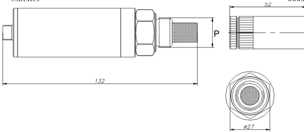
Рисунок 3.4 Внешний вид измерительного преобразователя ИПБТ-08
